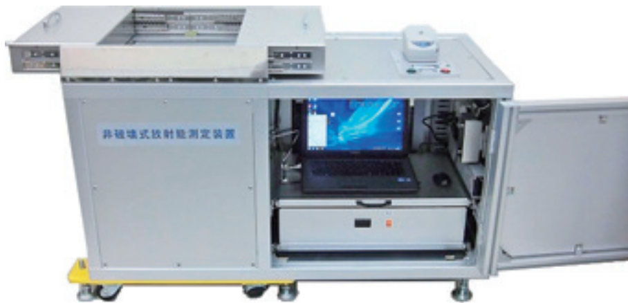
非破壊式放射能測定装置
